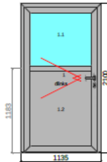
0014, Nebeneingang Hausmeister Menge: 1 Stück
