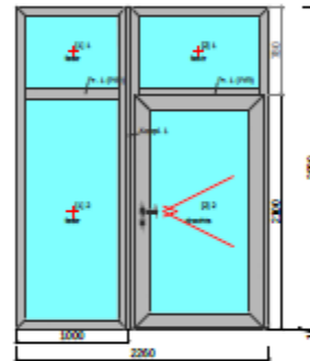
0015, Notausgangstür Treppenturm Menge: 1 Stück
