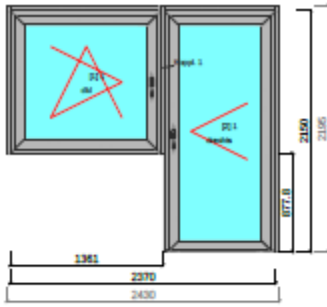
0010, Fenster/Türelement Nebeneingang Keller Menge: 1 Stück
