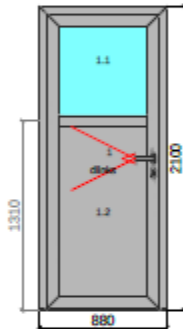
0013, [1] 1-teilige Haustür Menge: 1 Stück
